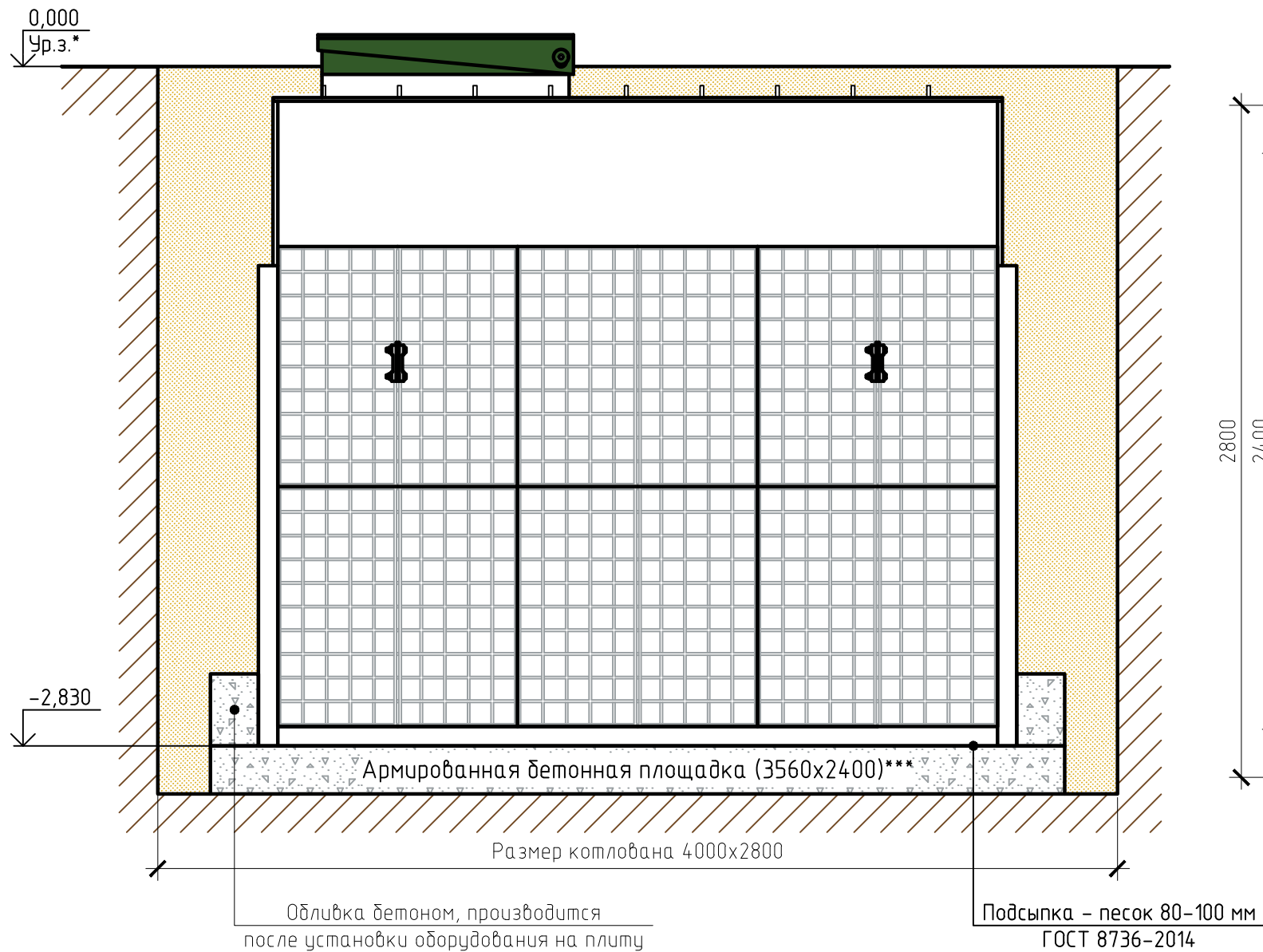
Вид спереди
